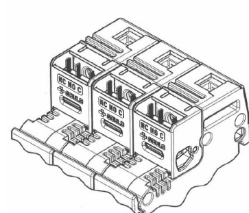
3 contacts auxiliaires Indépendants 3 x CMS14W1
