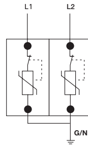
Phase divisée 2-Pôle - 3-Fils
